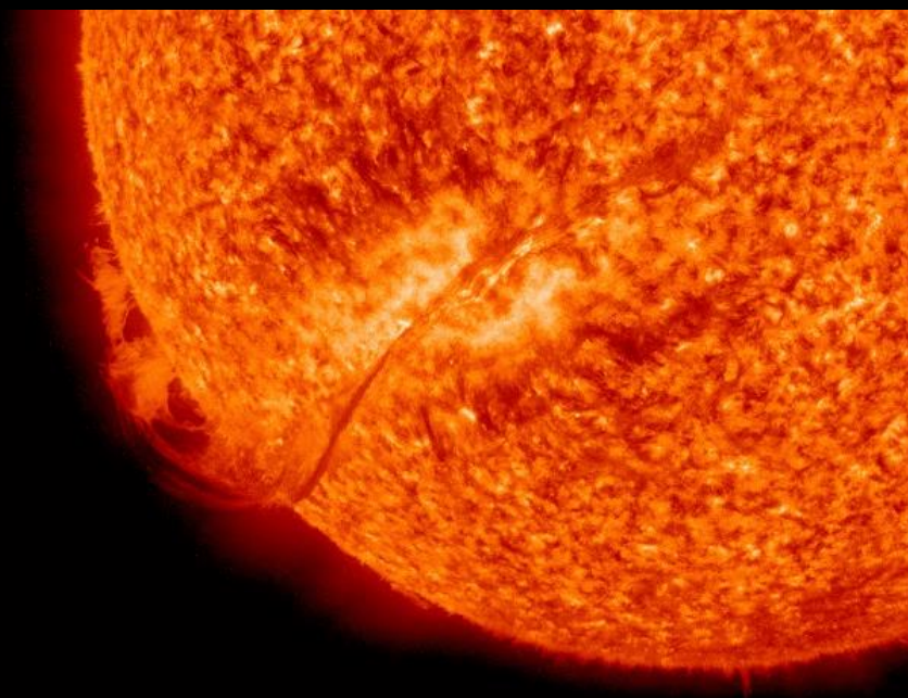
SDO/AIA 304 2010-12-06 14:35:33 UT
